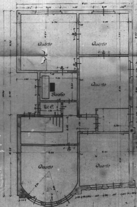
Planta baixa do andar primeiro
