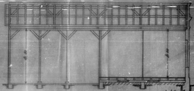
Corte longitudinal. f. 50.
