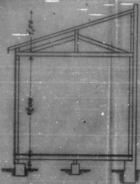
Corte transversal. f. 50.
