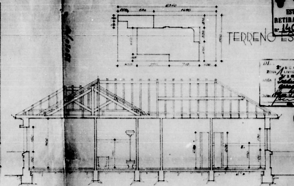
CORTE C-D
