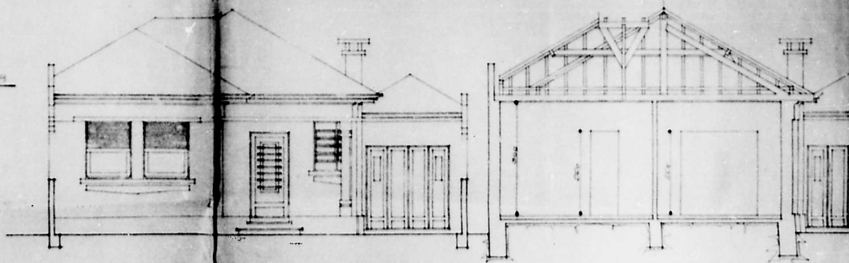
FACHADA
