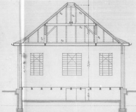
Corte longitudinal C-D
