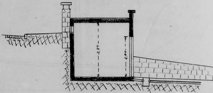
CORTE TRASVERSAL ESC 1:50
