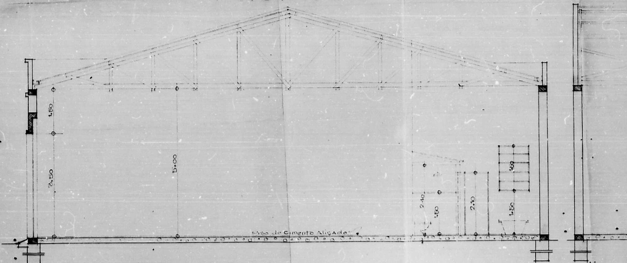
CORTE C-D
