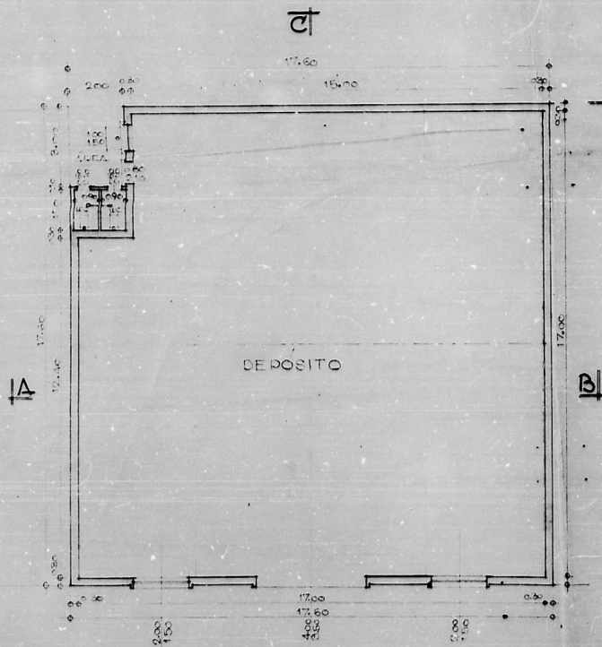
PLANTA BAIXA
