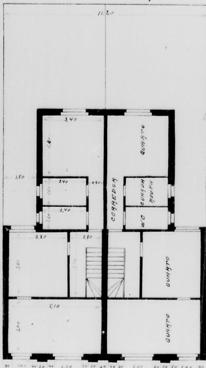
PLANTA BAIXA ESC 1:100 ANDAR SUPERIOR
