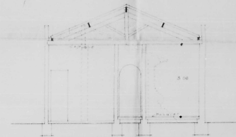
~ CORTE TRANSVERSAL ~
