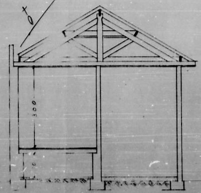
CORTE A-A 1/50
