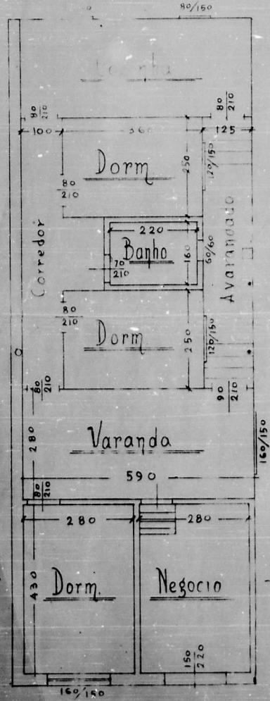
P. BAIXA 1/50
