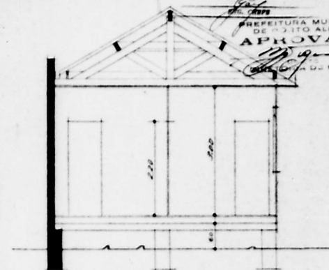
CÓRTE A-A
