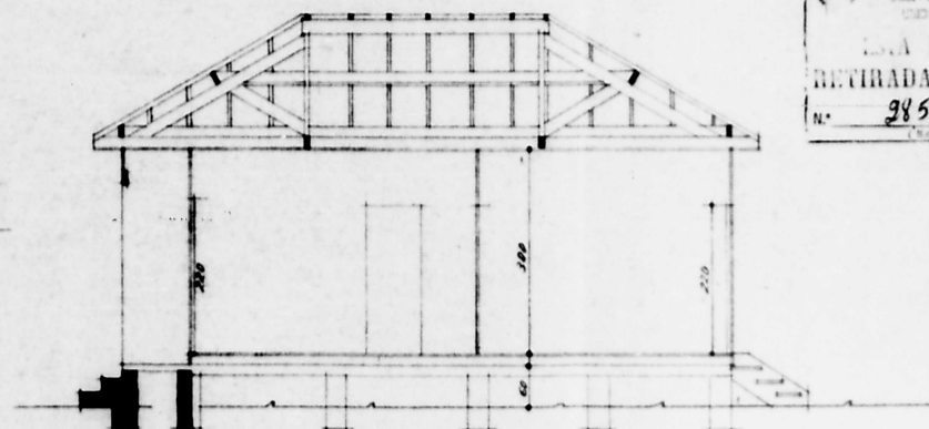
CÓRTE B-B
