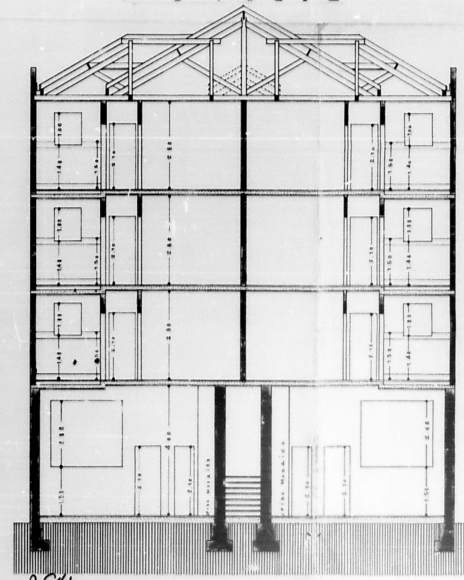
CORTA A-B
