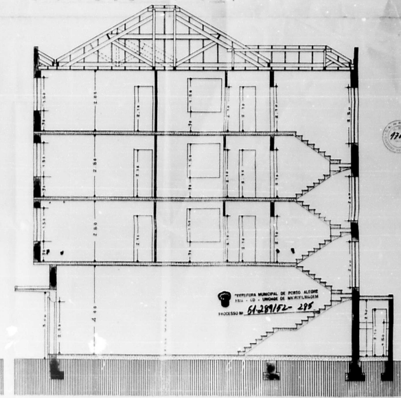
CORTA C-D
