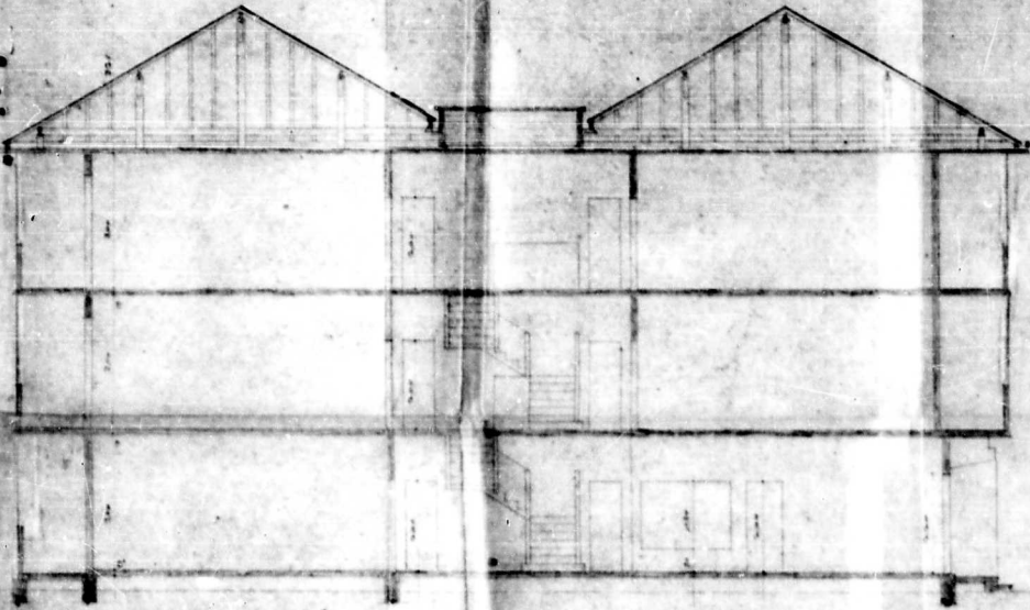
Corte Transversal
