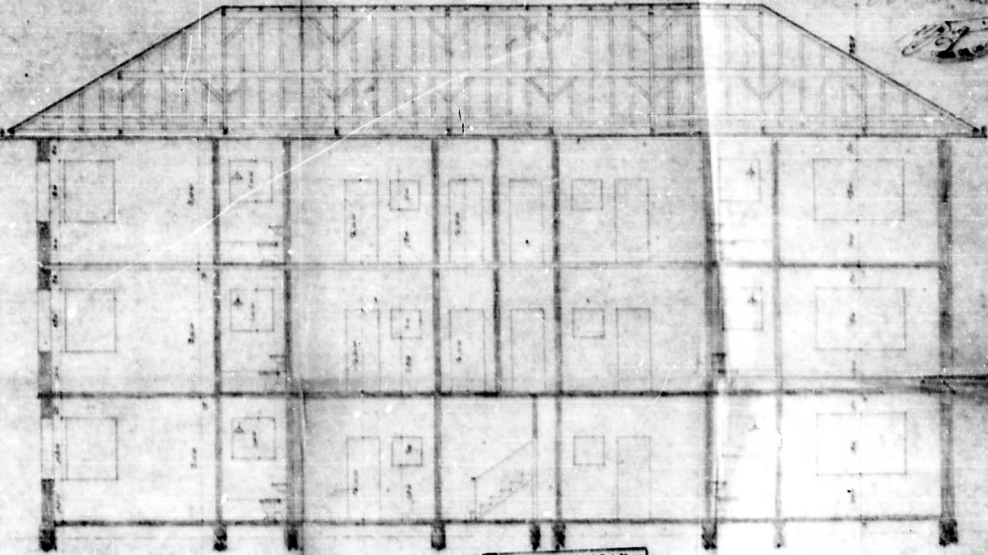
Corte Longitudinal
