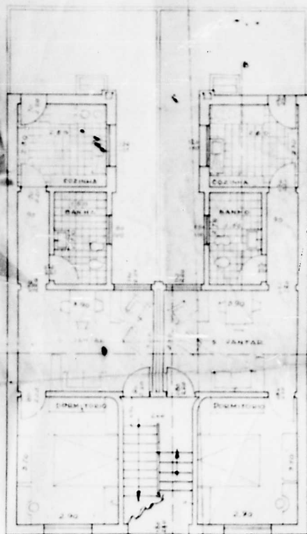
PLANTA TERREA
