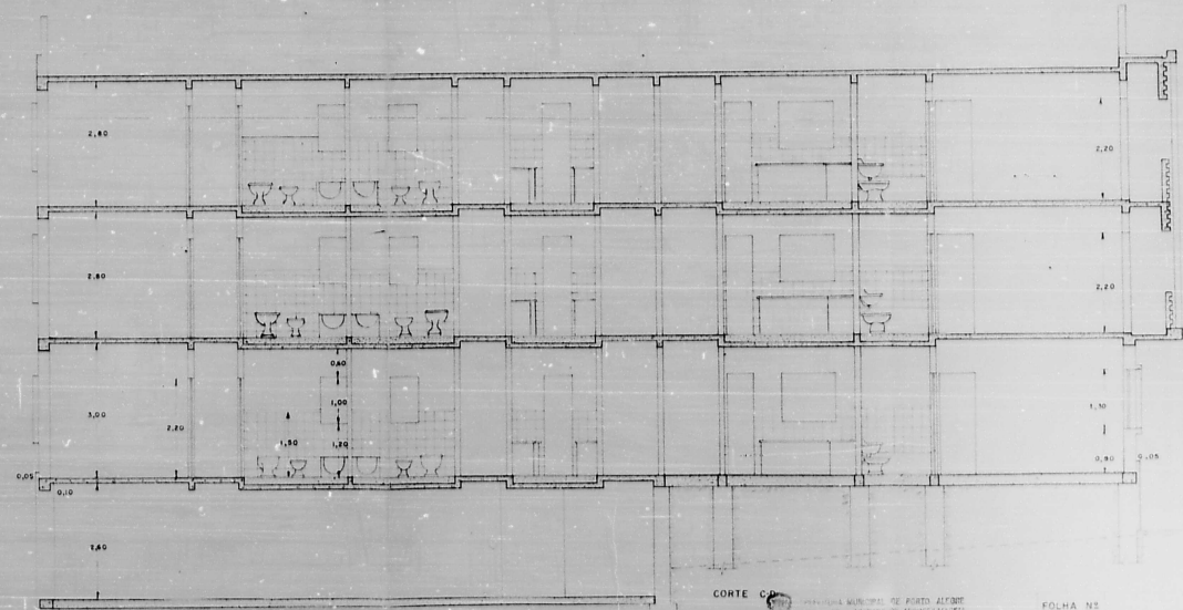
CORTE CA
