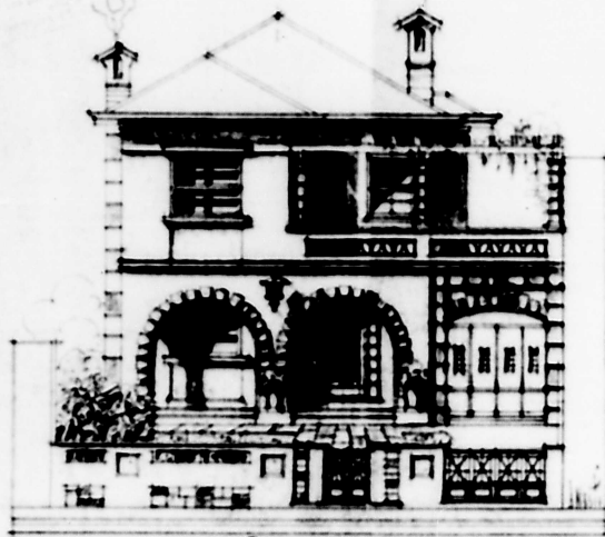
Fachada
