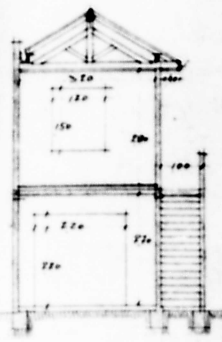
Corte B-B
