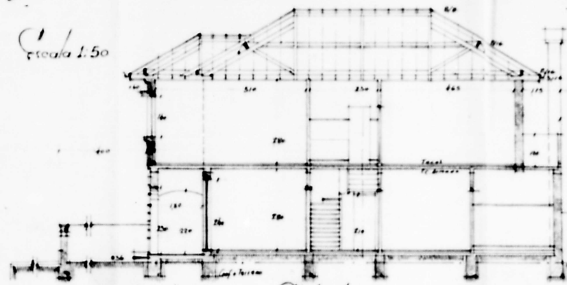
Corte A-B
