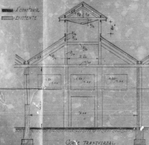
CORTE TRANSVERSAL 1:50
