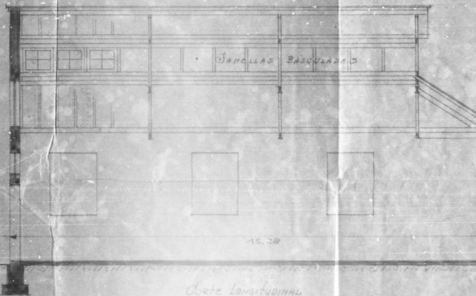
CORTE LONGITUDINAL 1:50
