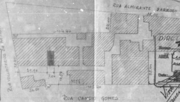
SITUAÇÃO 1:1000
