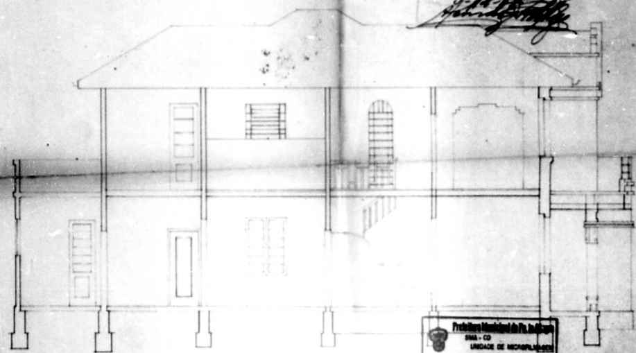
CORTE LONGITUDINAL
