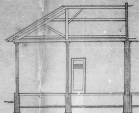
CÔRTE A/B
