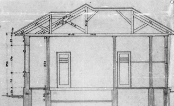
CÔRTE C/D
