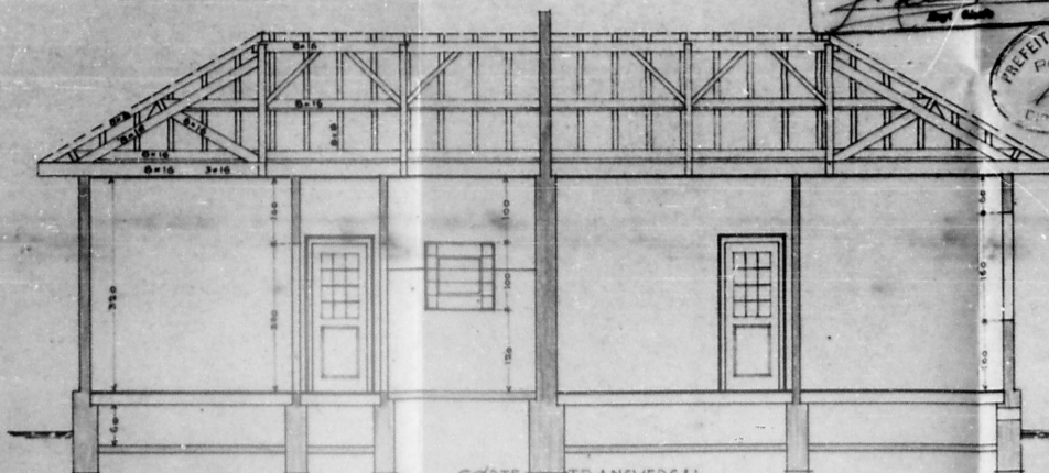
CORTE TRANSVERSAL
