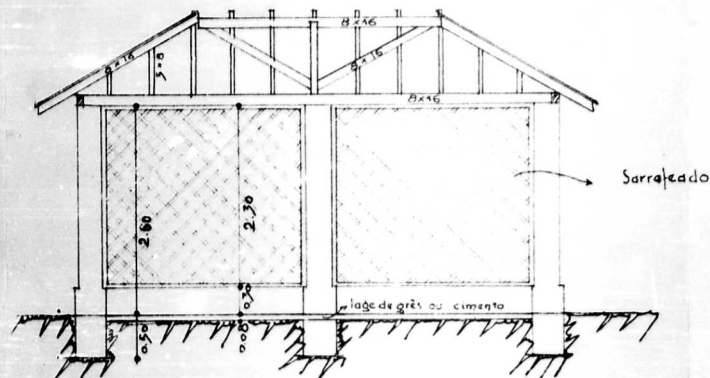
CORTE a-b
