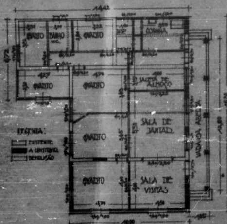
PLANTA - ESCALA 1:100
