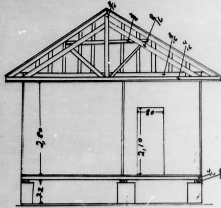
CORTE A.B. 1.50
