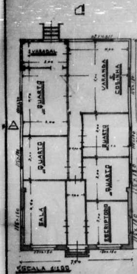
ESCALA 1:50
