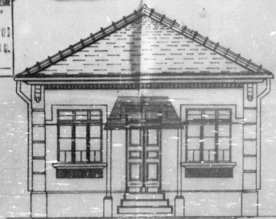
FRONTE
