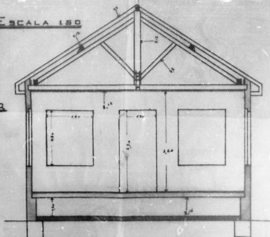
CORTE AB
