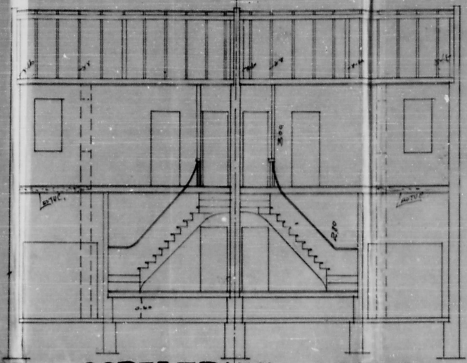
CORTE TRANSV. ESC 1:50
