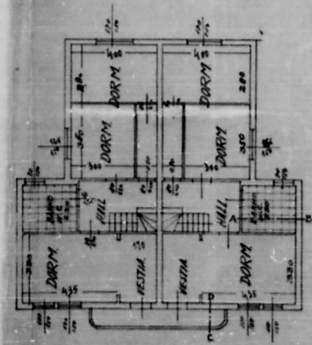
PAV. SUP. ESC. 1:100
