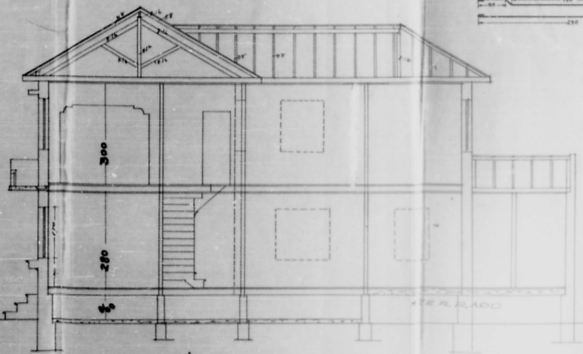
CORTE LONG. ESC 1:50
