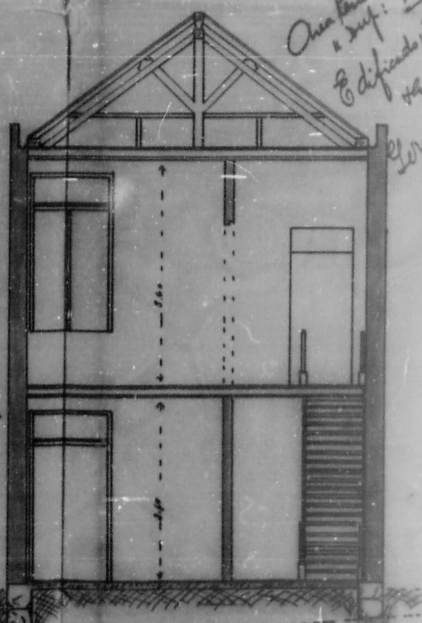
CORTE TRANSVERSAL 1.50
