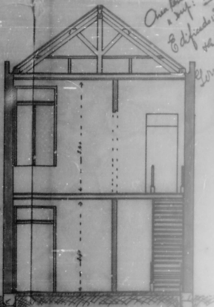
CORTE TRANSVERSAL 1:50
