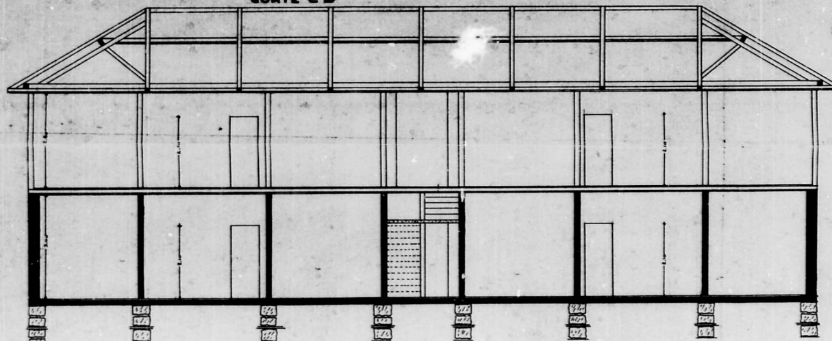
CORTE C-D
