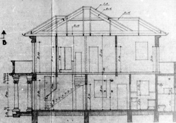
CORTE B-B
