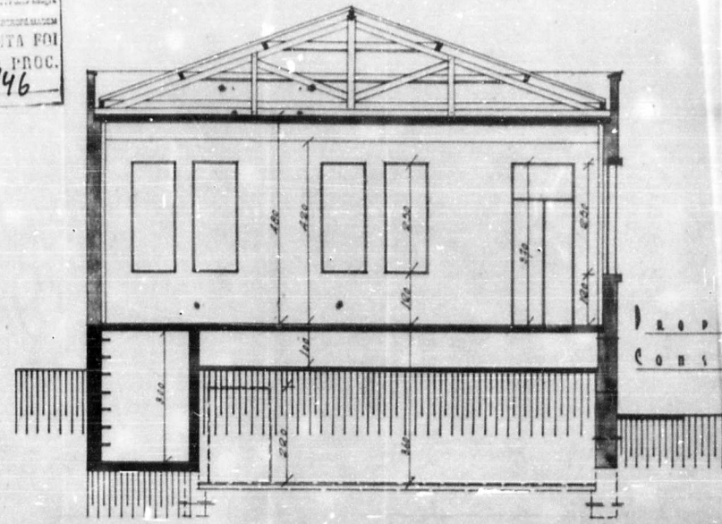
CORTE C-D
