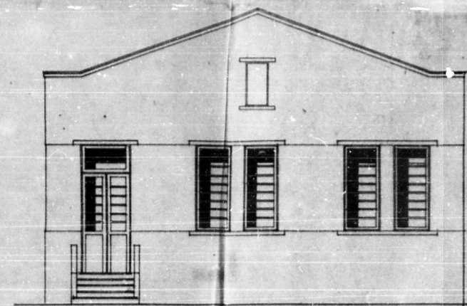
ELEVAÇÃO POSTERIOR
