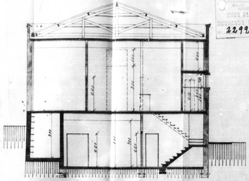
CORTE A-B
