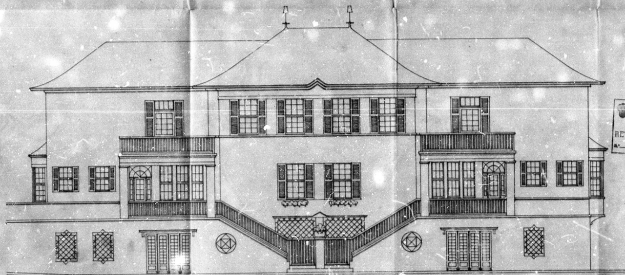
Fachada das casas á Praça São Manoel
