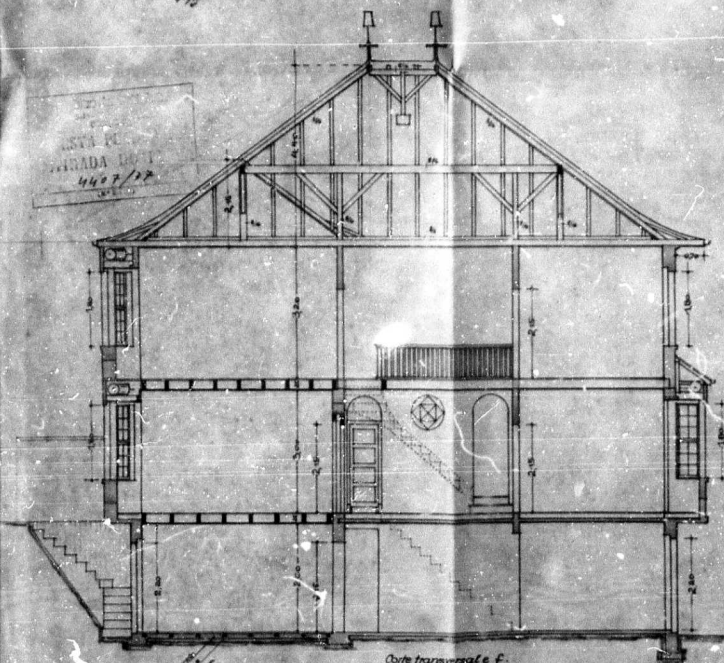
Corte transversal e-f das casas de Rua Dinarte Ribeiro e Tobias da Silva
