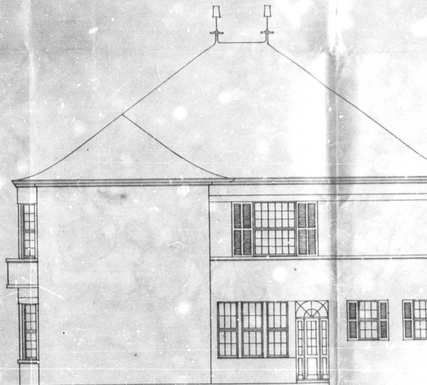
Fachada lateral das casas ás ruas Dinarte Ribeiro e Tobias da Silva
