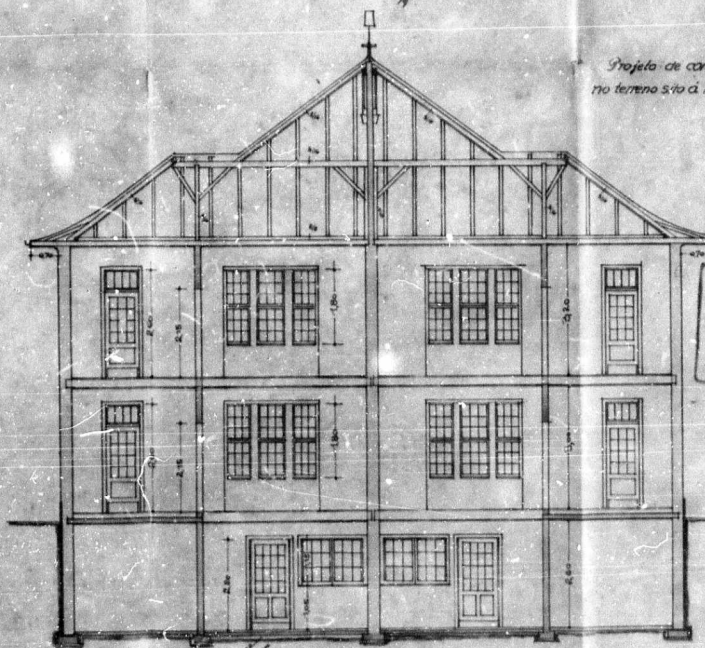
Corte longitudinal g-h das casas de Rua Dinarte Ribeiro e Tobias da Silva
