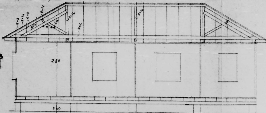
CORTE CD 1,50
