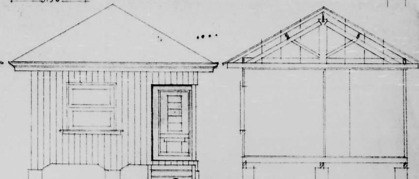
FRONTE 1,50
