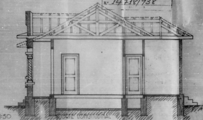
CORT. LONGITUDINAL
