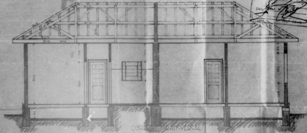
CORT. TRANSVERSAL
