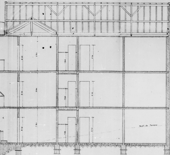
CORTE-AA-150
