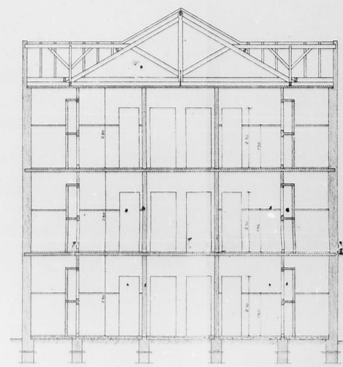
CORTE BB-1:50
