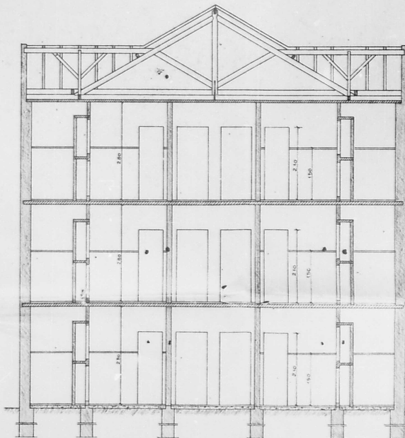
CORTE-BB-150
