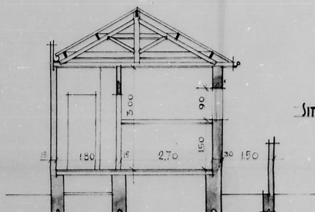
CORTE TRANSVERSAL 1:50
