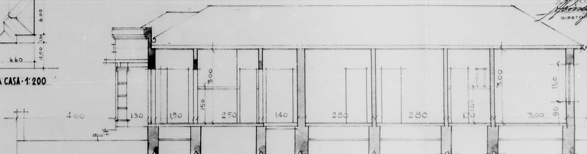
CORTE LONGITUDINAL 1:50
