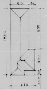
SITUAÇÃO DA CASA 1:200
