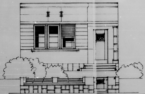
VISTA 1:50
