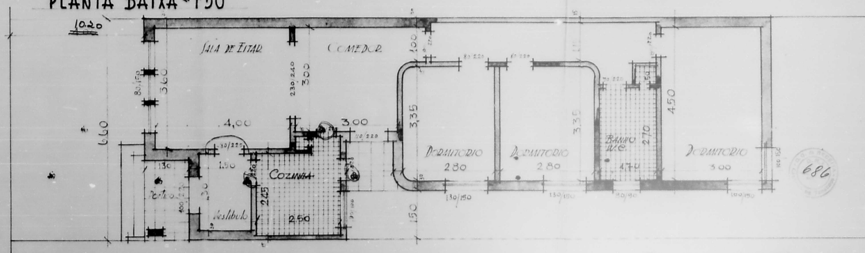
PLANTA BAIXA 1:50
