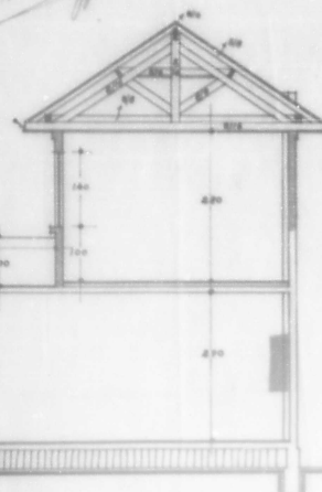
CORTE A.S. 1:50
