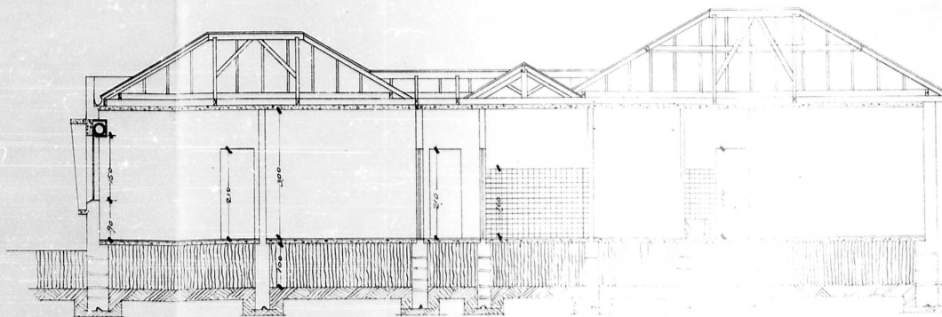
CORTE C-D
