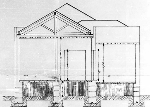
CORTE A-B
