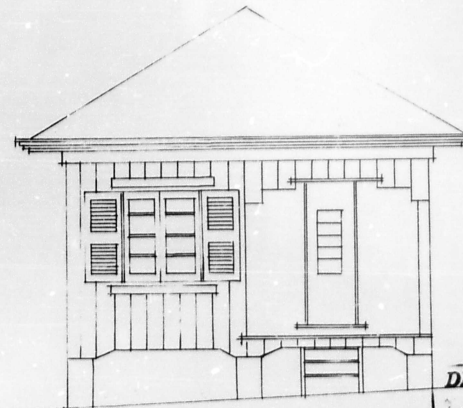
FACHADA 1/50
