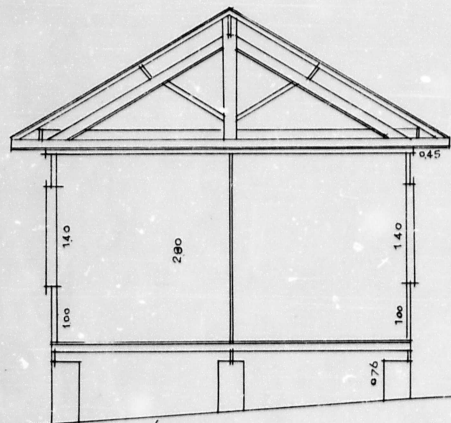
CORTE A-B ESCALA 1/50
