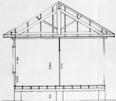
CORTE C-D
