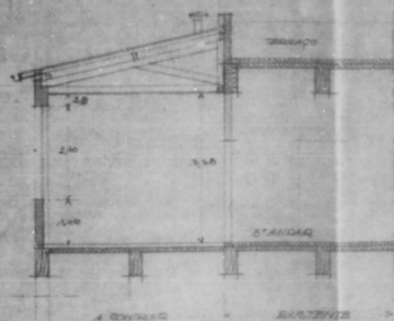
CORTE: A-B
