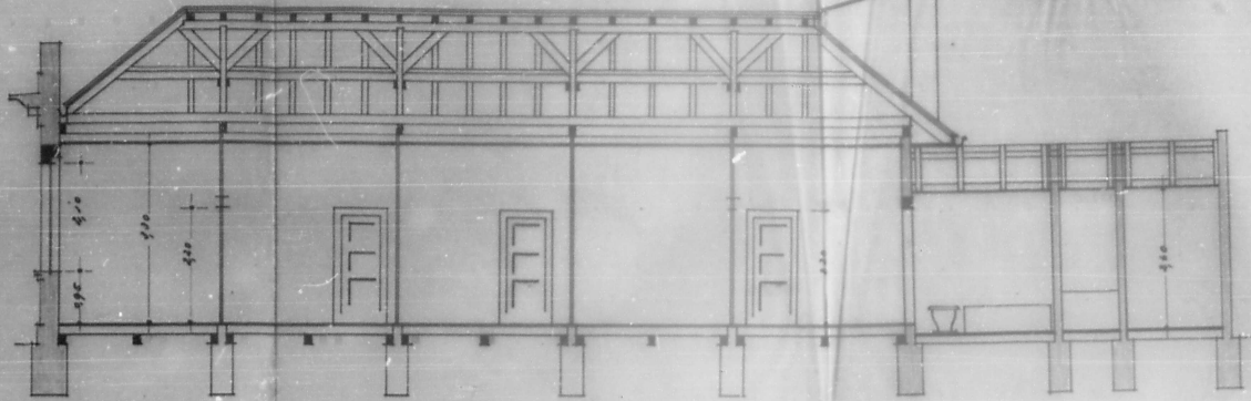
CORTE LONGITUDINAL
