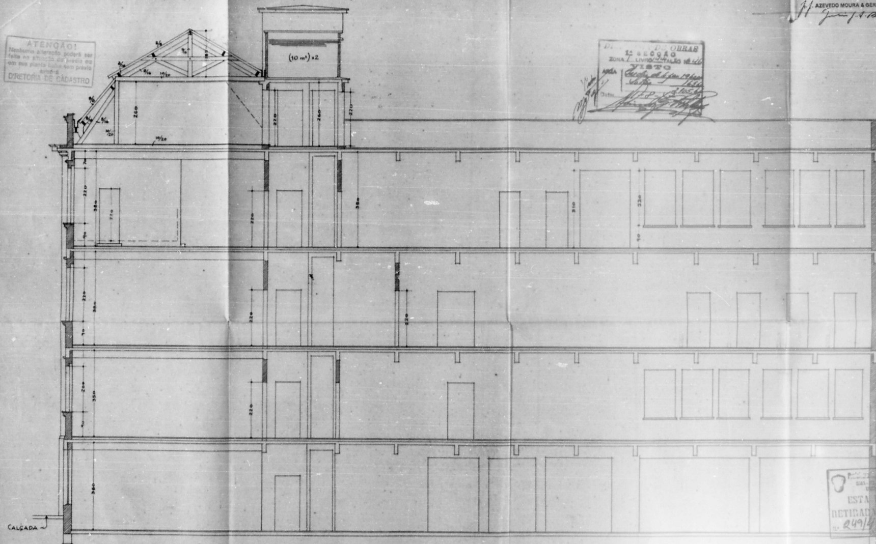
CORTE C-D
