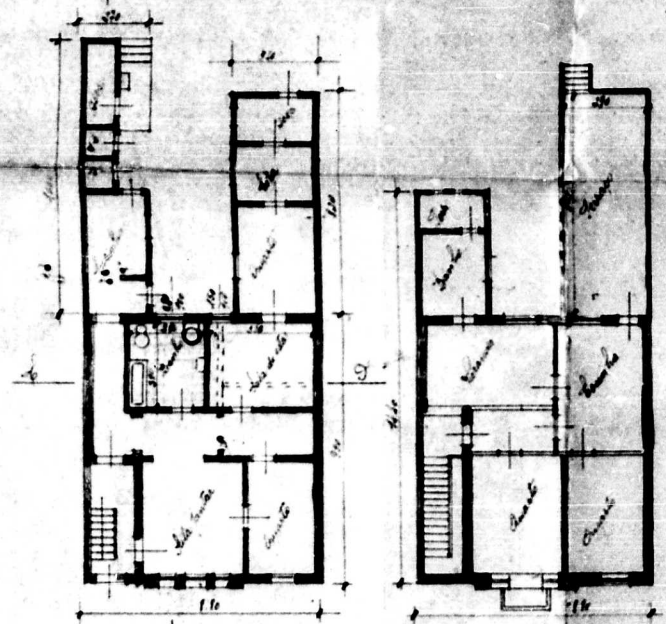
PLANTA BAIXA Esc. 1:100
