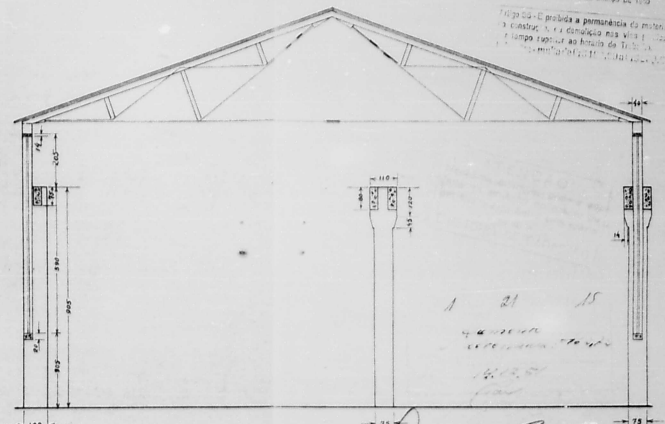
Corte B-B
