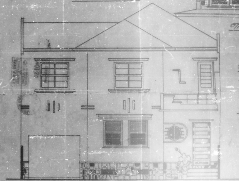
Fronte-150
