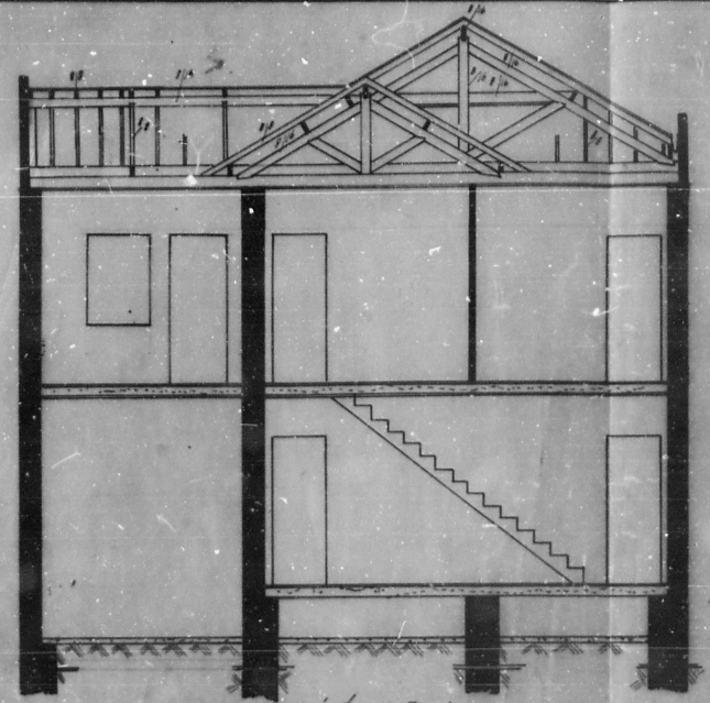
Corte A-B-150
