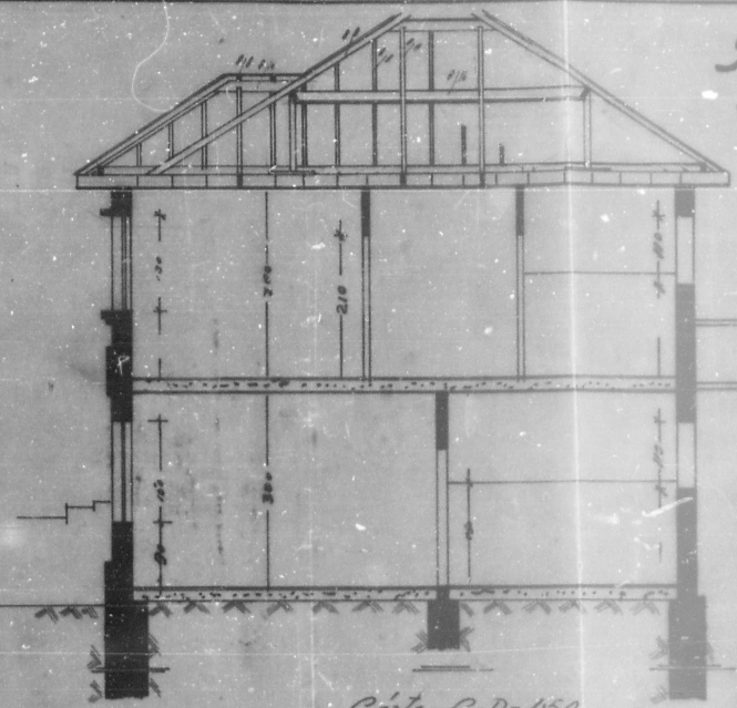
Corte C-D-150
