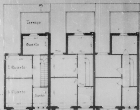
Andar superior.
