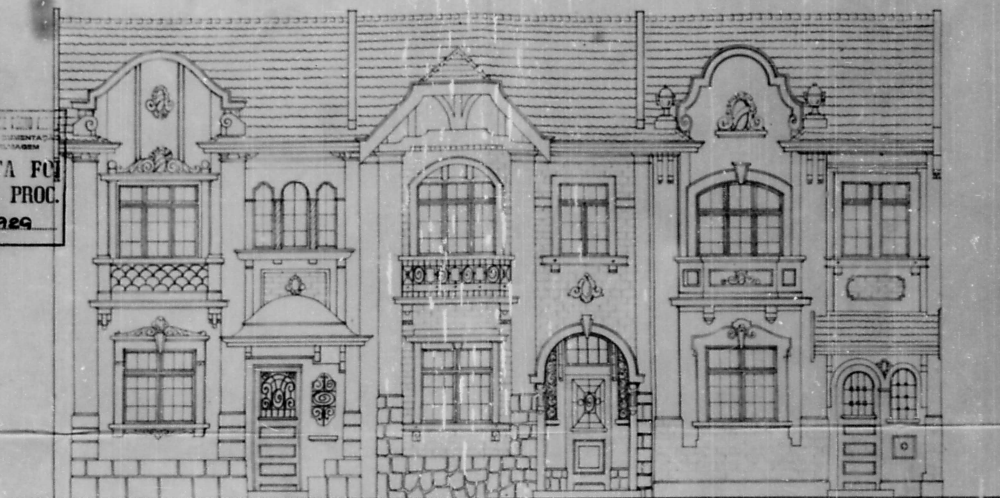
Fa.çada - 1:50.
