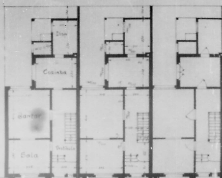
Andar térreo
