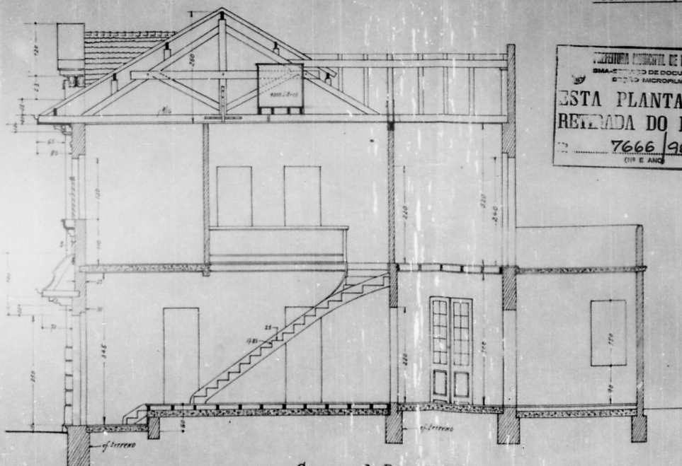
Corte - A-B - 1:50.
