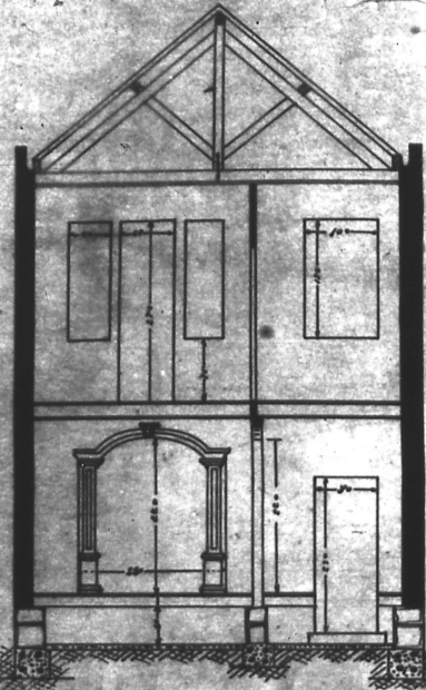
— CÔRTE TRANSVERSA —
