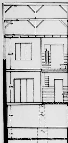
CORTE A-B 1:50
