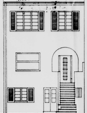
FACHADA 1:50
