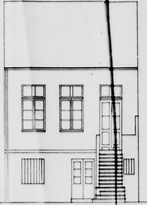
FACHADA 1:50 EXISTENTE
