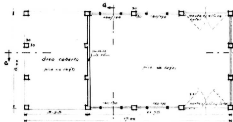
PLANTA 1:100
