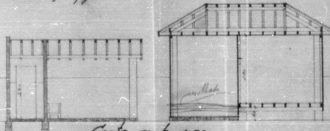
Corte a-b. 1:50
