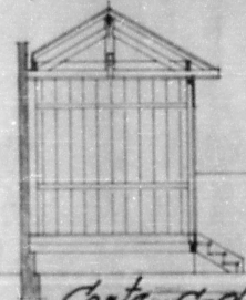
Corte c-d. 1:50
