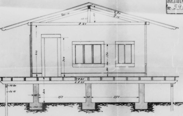
CORTE
