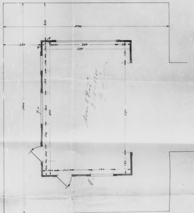
PLANTA BAIXA
