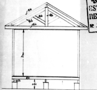
Cortes Esc. 1:50
