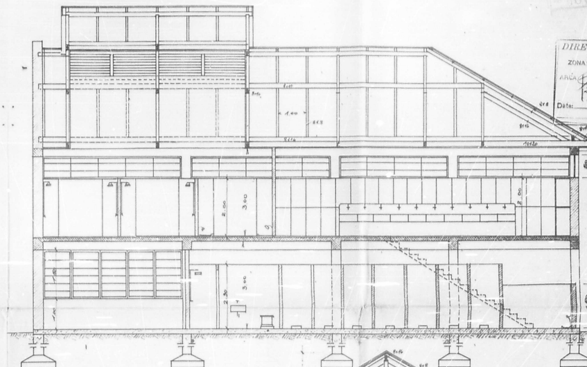
CORTE LONGITUD.
