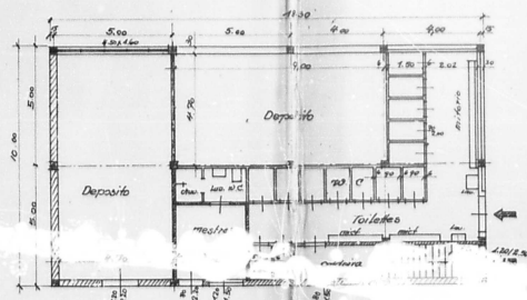
ANDAR TERREO
