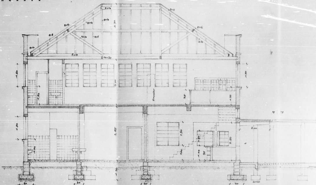
CORTE LONGITUDINAL
