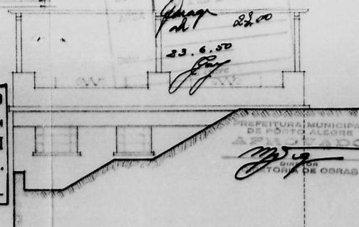
FACHADA LATERAL
