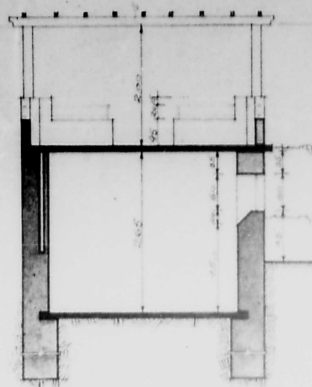
CORTA TRANSVERSA
