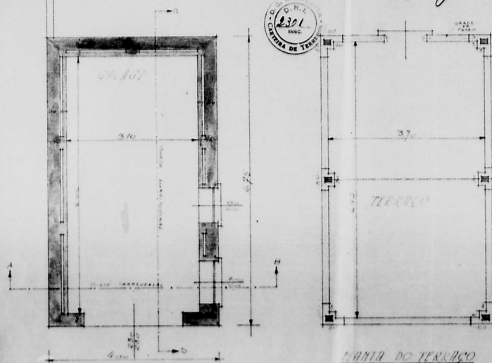
PLANTA BAIXA
